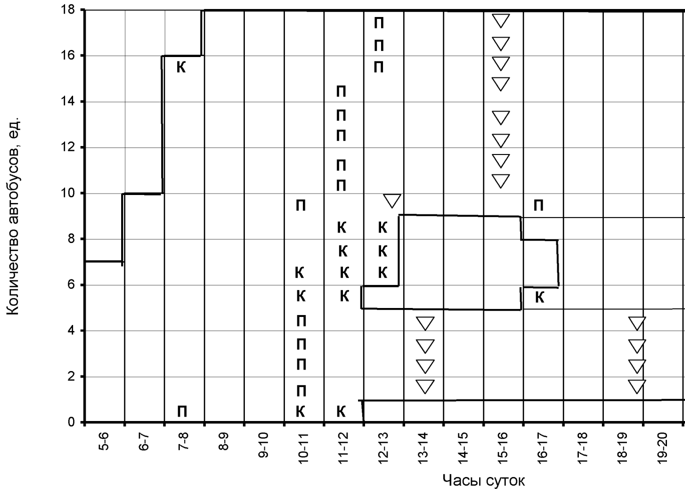
Рисунок 5. Окончательный вариант распределения автобусов по часам суток и определение сменности их работы
