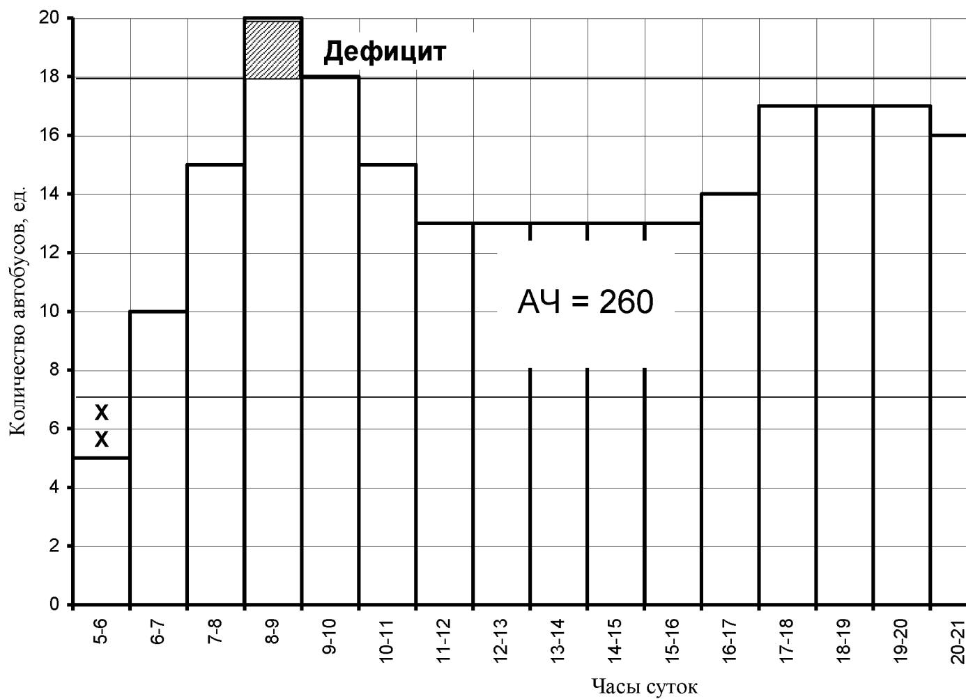
Рисунок 3. Расчетное распределение автобусов по часам суток
