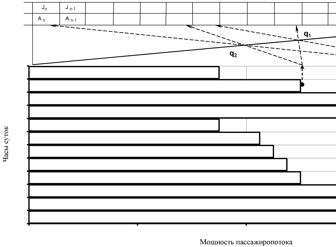
Рисунок 1. Номограмма для определения потребного количества автобусов на маршруте по часам суток
