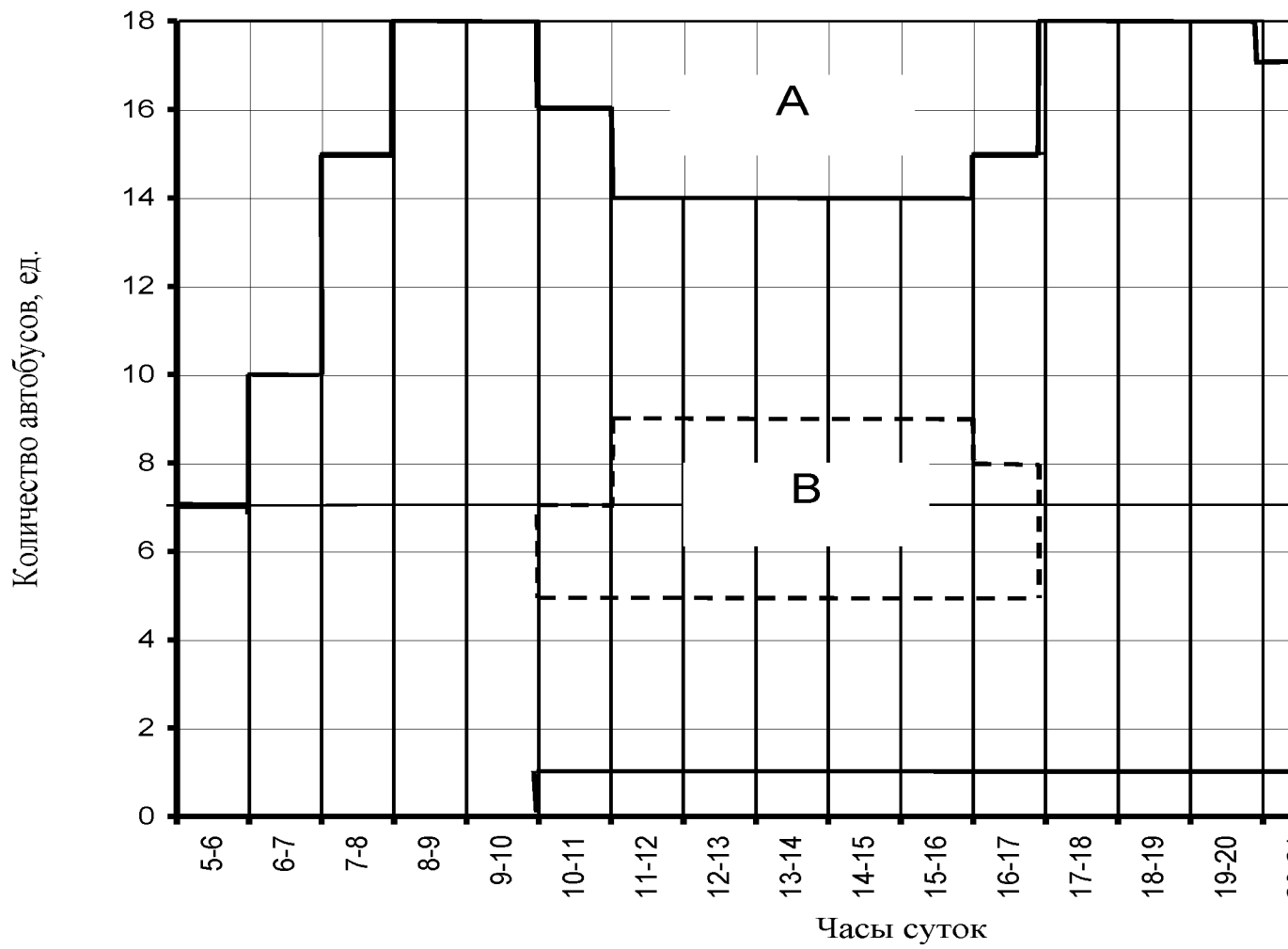
Рисунок 4. Промежуточный вариант распределения автобусов по часам суток
