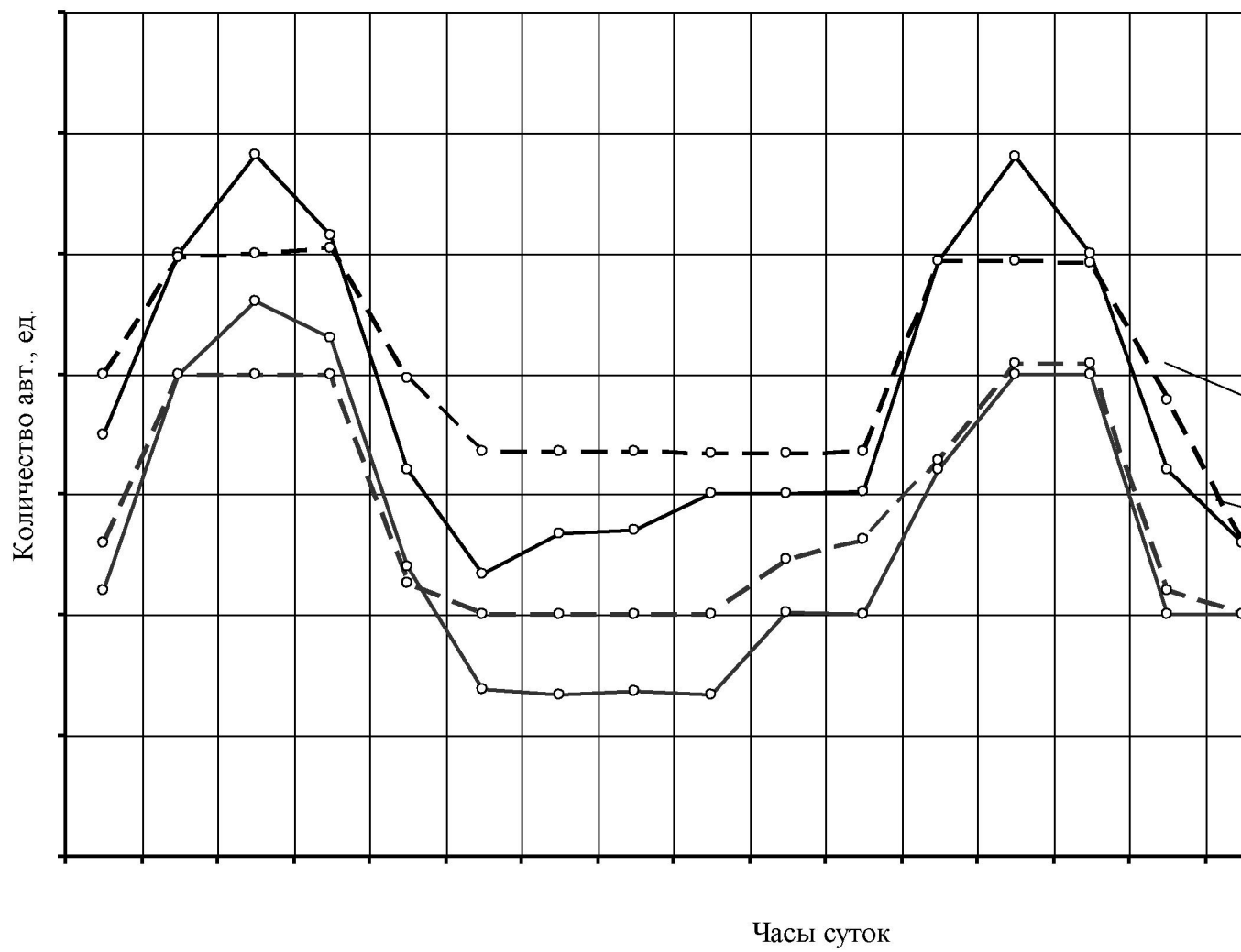
Рисунок 2. Корректировка выпуска автобусов на маршрут по часам суток
