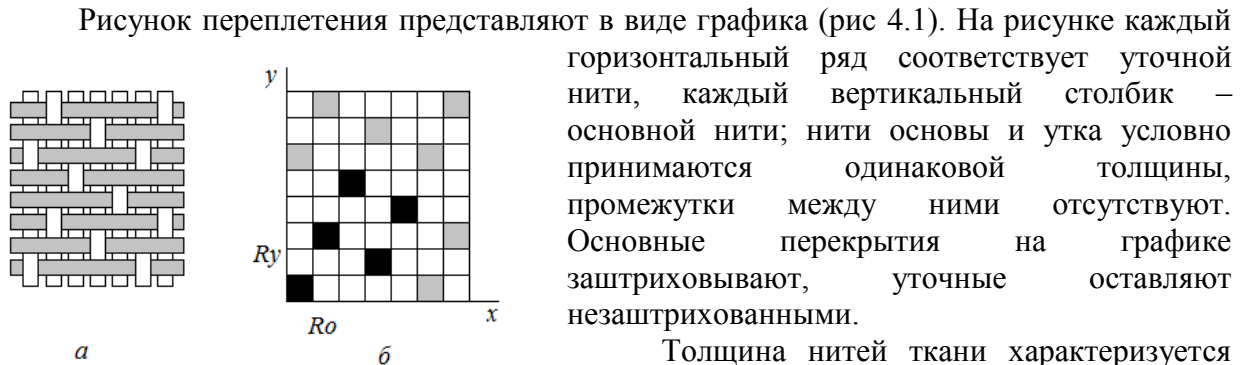
Рисунок 4.1 – Схема (а) и график (б) ткацкого переплетения
