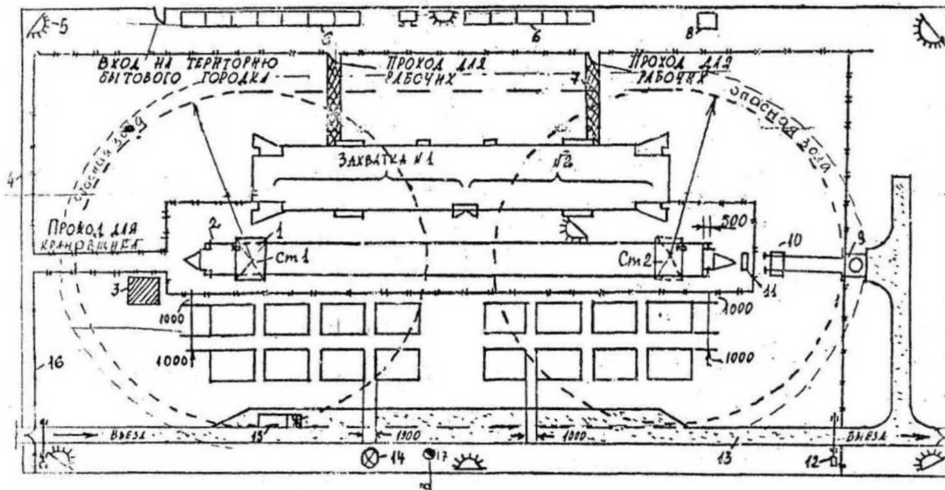
Рисунок 2 - Безопасная организация строительной площадки при возведении надземной части здания: 1 - башенный кран; 2 - тупиковый упор; 3 - место для хранения съемных грузозахватных приспособлений и тары; 4 - инвентарное защитноохранное ограждение; 5 - осветительная вышка с прожекторами; 6 - бытовое помещение; 7 - временные защитные козырьки; 8 - туалет; 9 - растворный узел; 10 - тележка для транспортировки раствора; 11 - контрольный груз; 12 - шлагбаум; 13 - временная дорога из сборных ж/б плит; 14 - место нахождения водителя; 15 - автомобиль; 16 - защитное ограждение; 17 - пожарный гидрант
