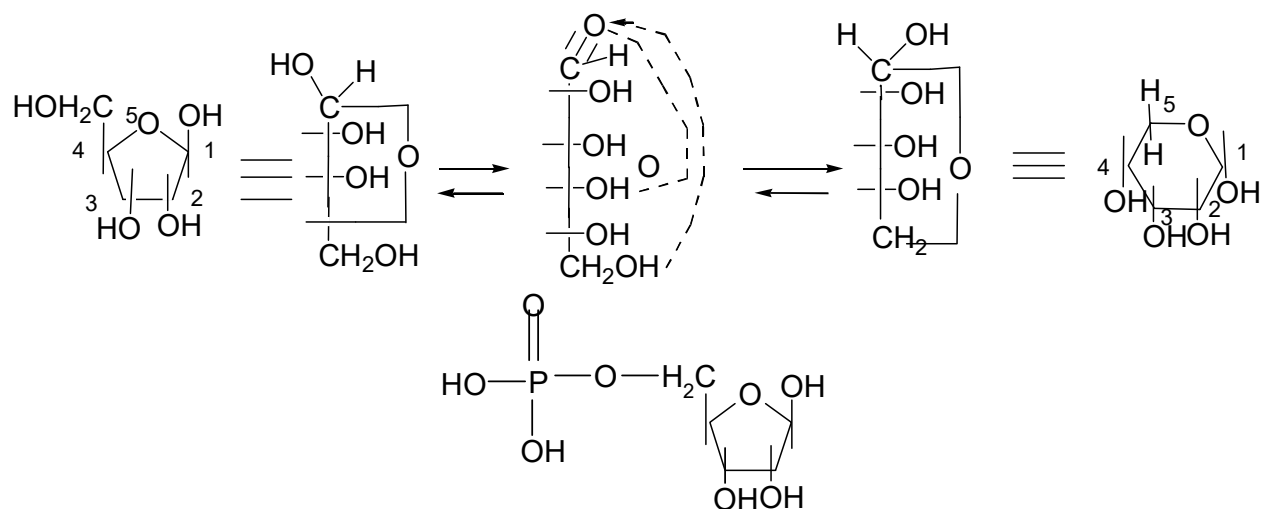
5-монофосфат \beta -D-рибофуранозы
