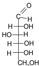
D-глюкоза
