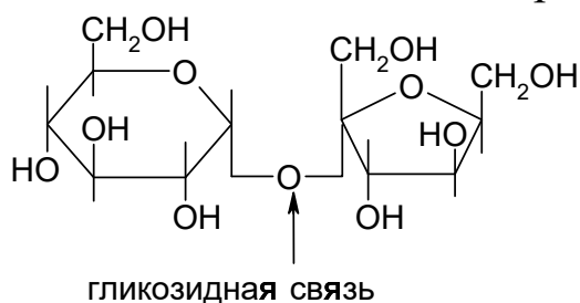
Сахароза
