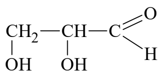
Глицериновый альдегид
