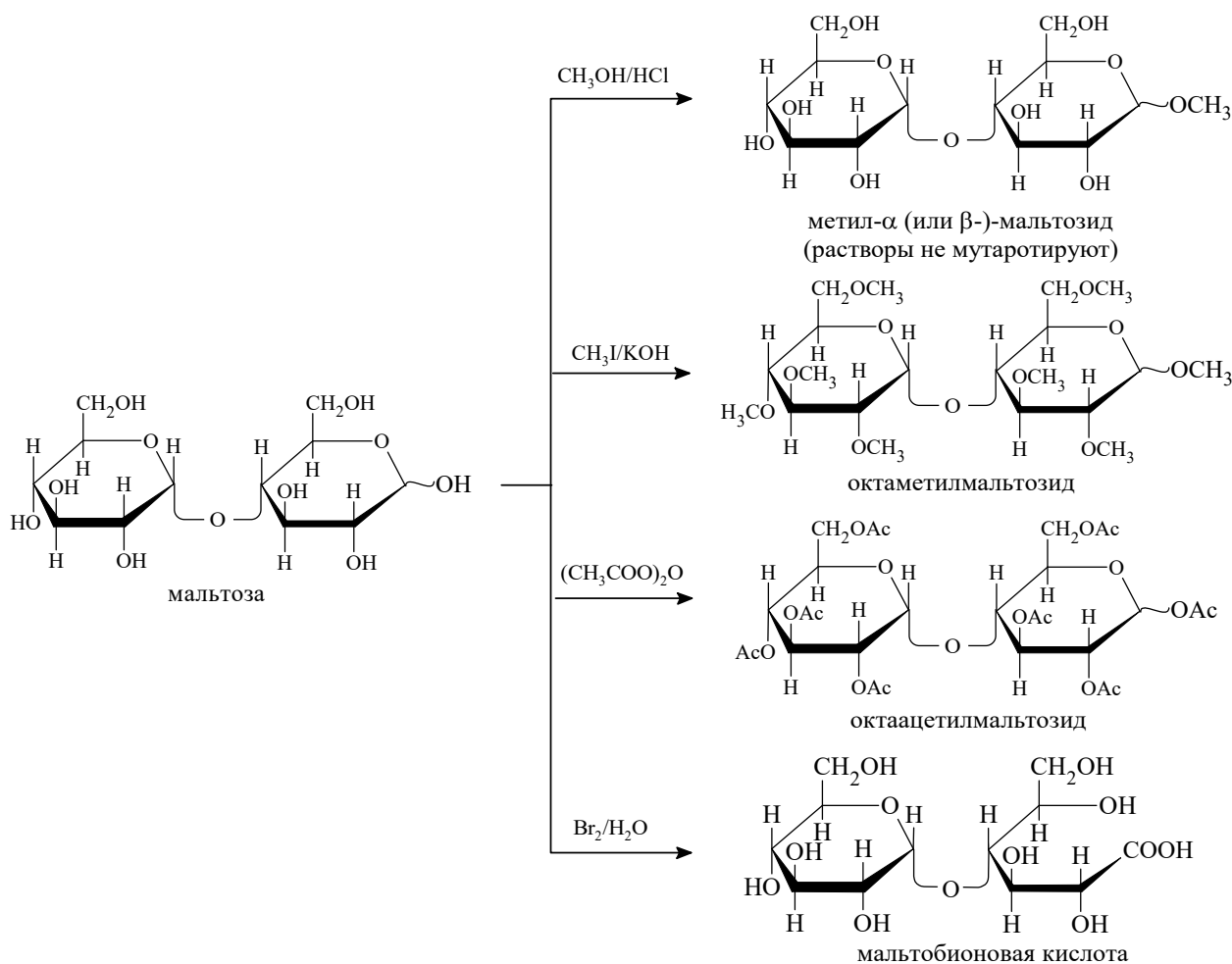
Схема 2. Химические превращения мальтозы
