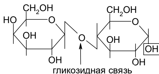
Лактоза
