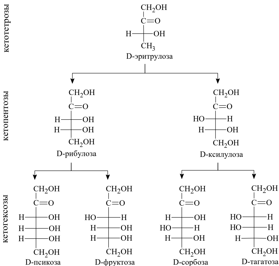
Рис. 2. Семейство D-кетоз.
