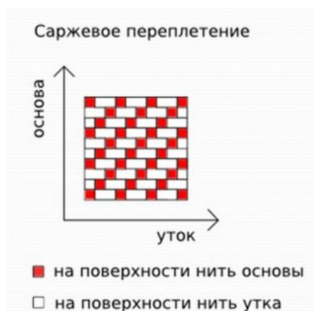
Рисунок 7 – Схема саржевого переплетения
