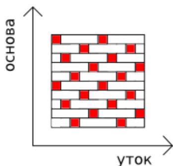
Сатиновое переплетение
