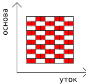
Поперечное репсовое переплетение
